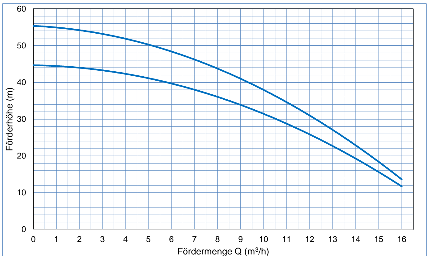
Kennliniendiagramm BWZ-80-S 16 ID
