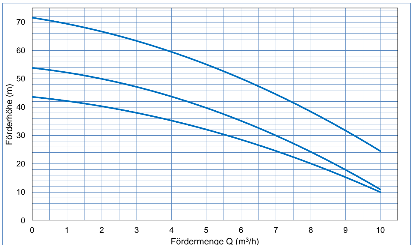
Kennliniendiagramm BWZ-80-S 10 ID
