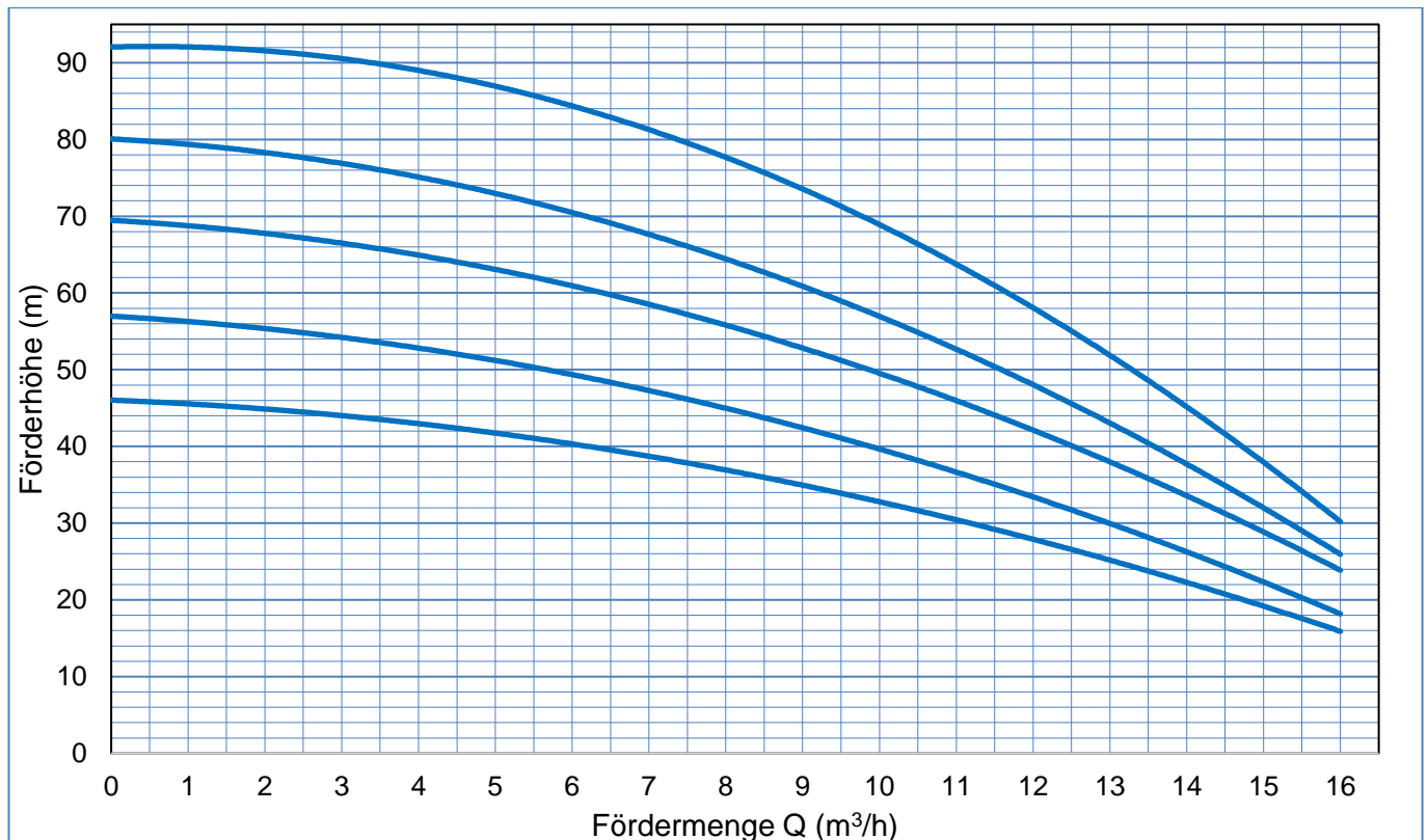
Kennliniendiagramm BWZ-160-H 16
