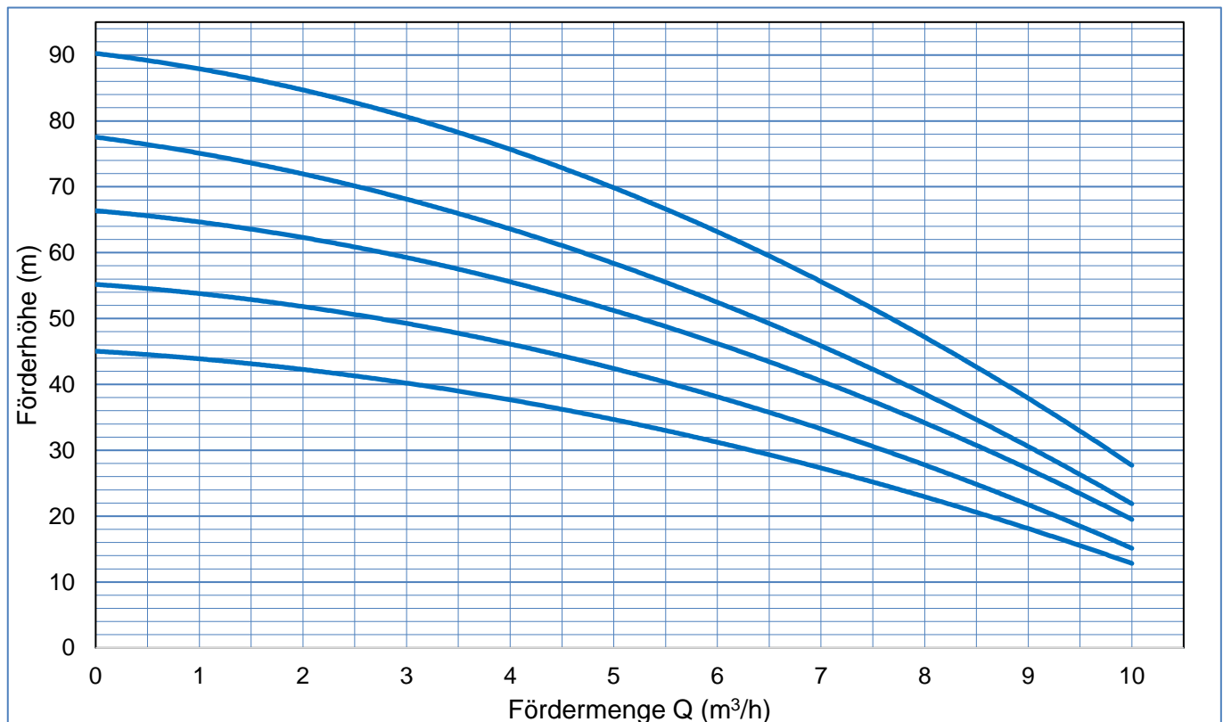
Kennliniendiagramm BWZ-160-H 10
