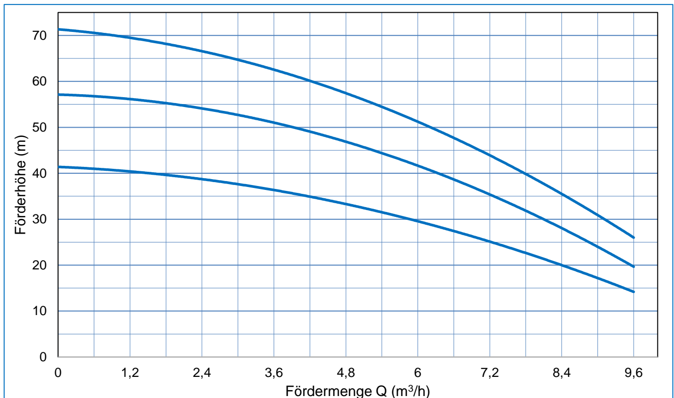
Kennliniendiagramm BWZ-80-D 10
