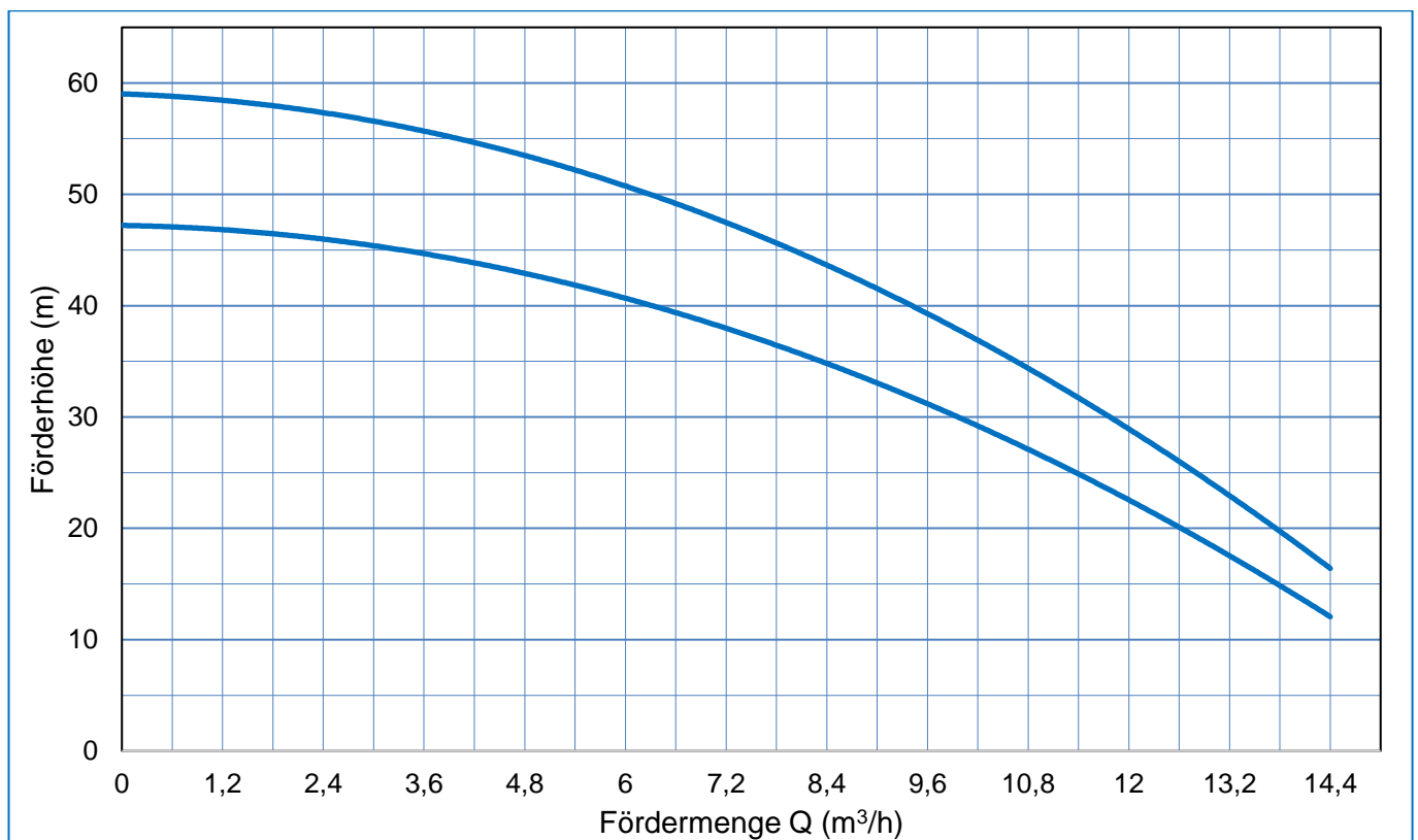
Kennliniendiagramm BWZ-80-D 14
