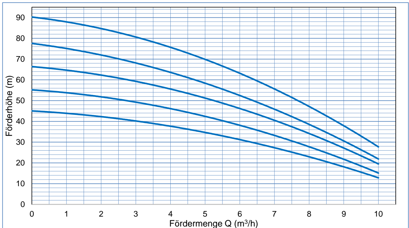
Kennliniendiagramm BWZ-160-H 10 SC
