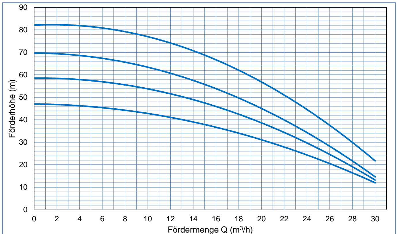
Kennliniendiagramm BWZ-160-H 30 SC
