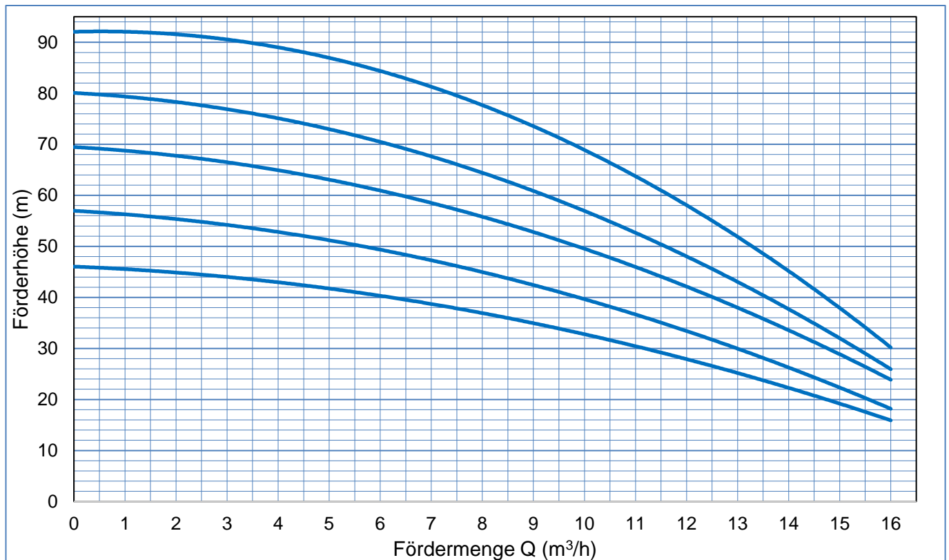
Kennliniendiagramm BWZ-160-H 16 SC
